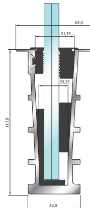
Perfil Central com furos escareados.
