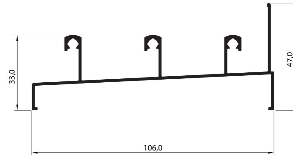
P-1258 Perfil SU 011 0,946 Kg/m
