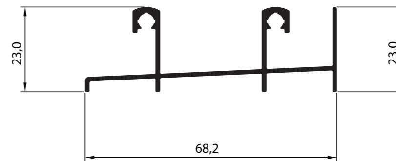
P-1286 Perfil SU 260 0,568 Kg/m
